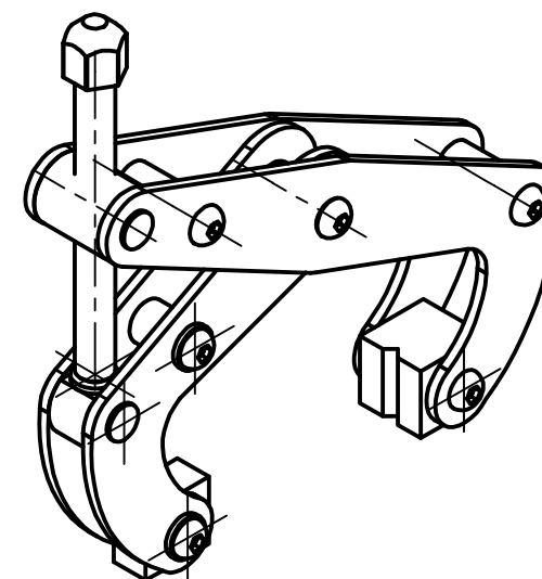
Аксонетрическая проекция
